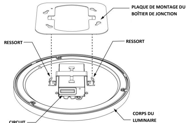
FIG. 3 (BOÎTIER DE JONCTION ET FILS RETIRÉS POUR PLUS DE CLARTÉ)
