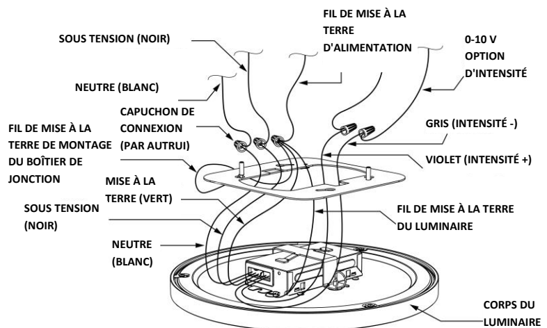
FIG. 2 (BOÎTIER DE JONCTION RETIRÉ POUR PLUS DE CLARTÉ)
