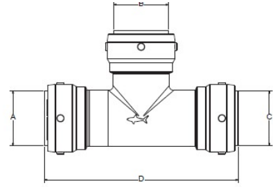
Tee
