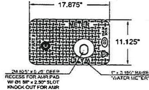
LID TOP VIEW
